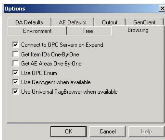
OPC DataSpy Browsing Options
