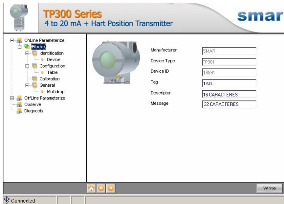
Figura 3 – Tela da Função “Online Parameterize” do TP301DTM
