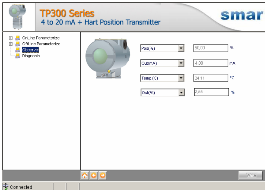
Figura 5 – Tela da Função “Observe” do TP301DTM
