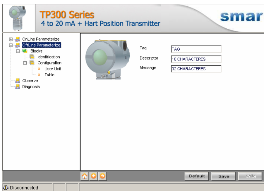
Figura 4 – Tela da Função “Offline Parameterize” do TP301DTM
