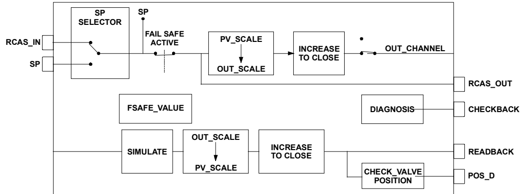
Figura 2.2 – Bloco de Saída Analógica
