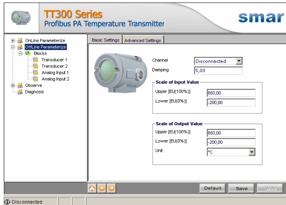
Figura 4 – Tela da Função “Offline Parameterize” do TT303DTM
