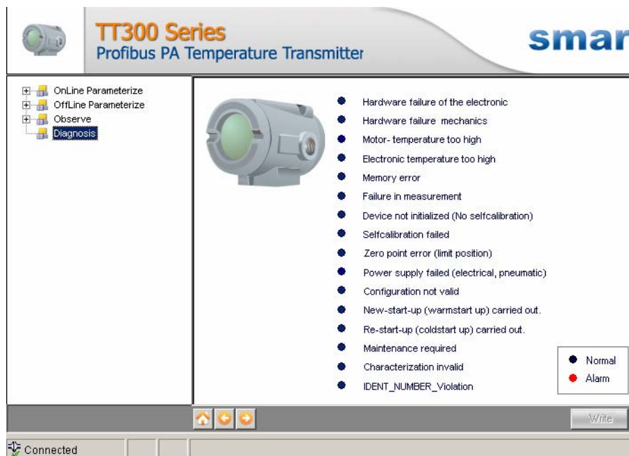
Figura 6 – Tela da Função “Diagnosis” do TT303DTM
