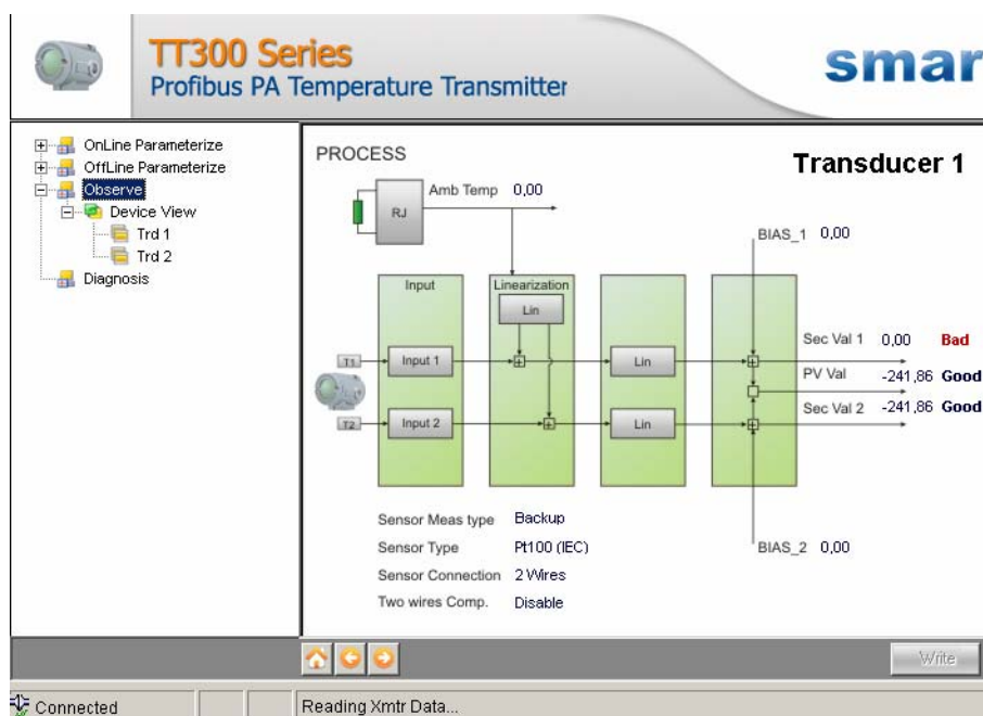
Figura 5 – Tela da Função “Observe” do TT303DTM
